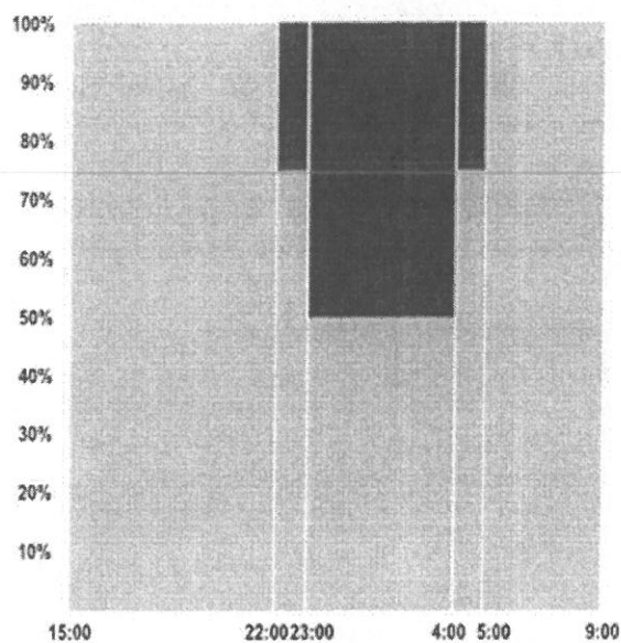
2. ábra: Fényáram szabályozás első változata
