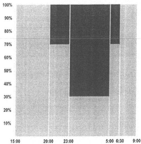
3. ábra: Fényáram szabályozás második változata
